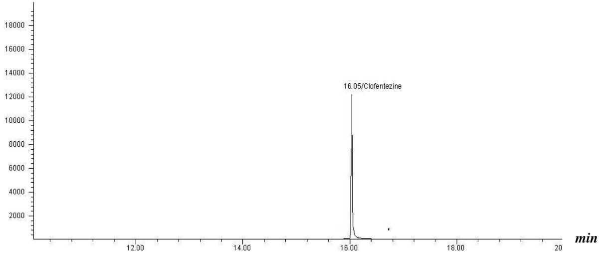
图 B.1 四螨嗪标准物质的气相色谱-质谱选择离子色谱图
