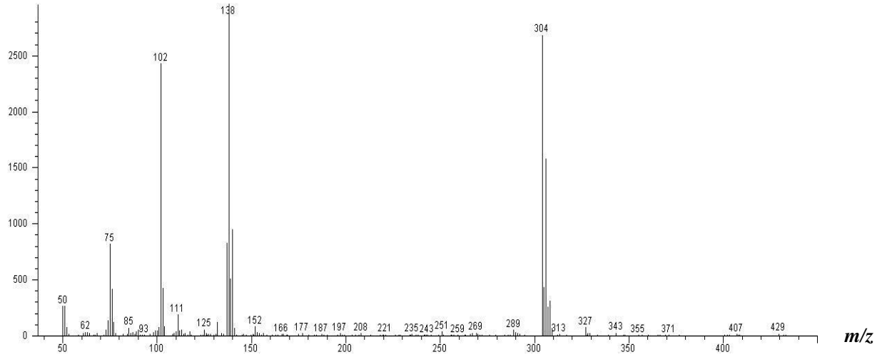
图 C.1 四螨嗪标准品的气相色谱-质谱图
